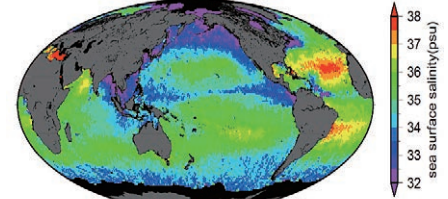
人工衛星による海面塩分 (Aquarius/SAC-D)
